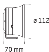
Afmetingen(mm) versterker type 620 en luidspreker type DKL600
